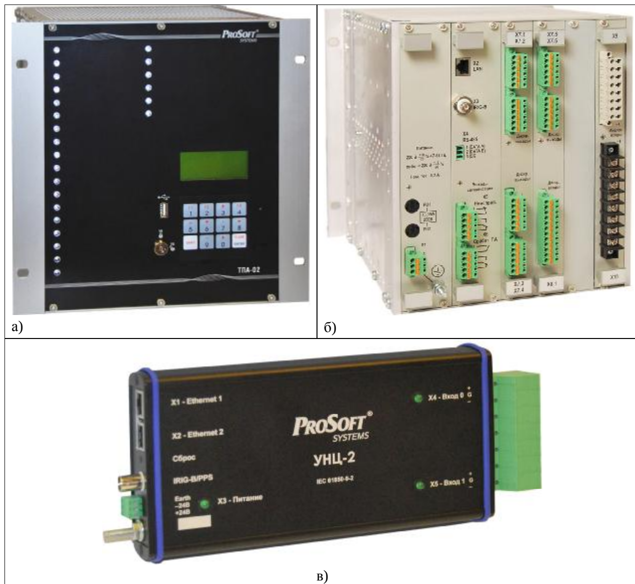
Рисунок 1. Внешний вид регистратора: а) главный вид; б) вид сзади; в) УНЦ-2.
